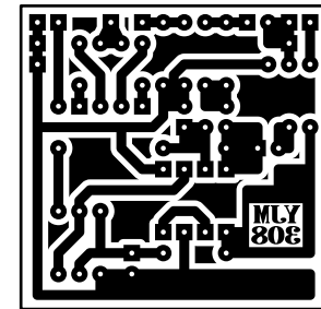
<実寸PCB>
